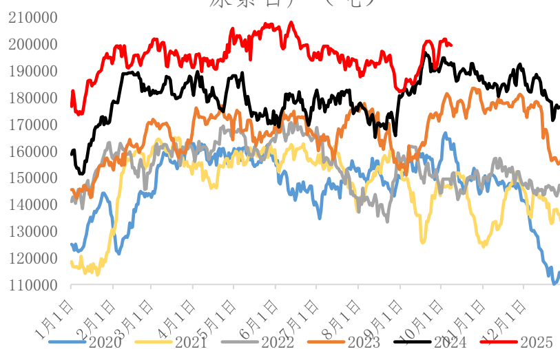
尿素日产（吨）
