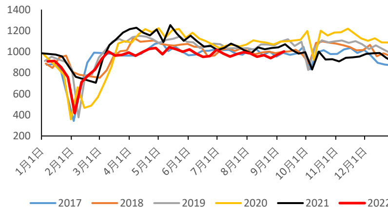
五大钢材表观消费量 (万吨)
