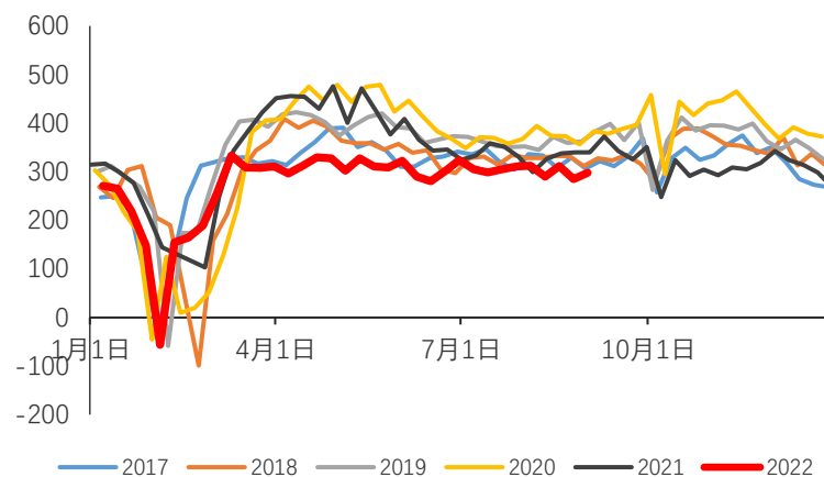
螺纹钢表观消费 (万吨)
