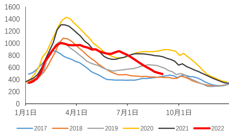
螺纹钢社会库存 (万吨)
