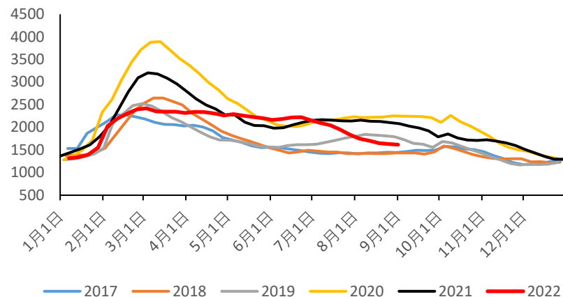
五大钢材总库存 (万吨)
