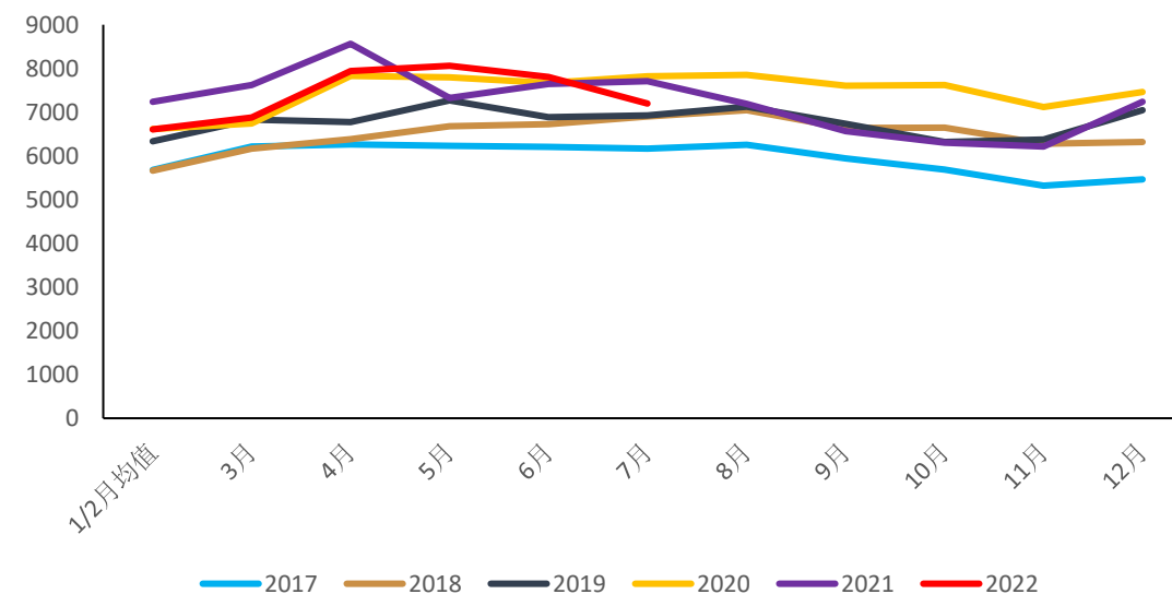
生铁产量：当月值：万吨
