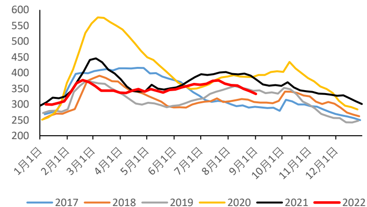
热轧卷板总库存（万吨）
