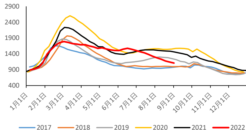
五大钢材社会库存 (万吨)
